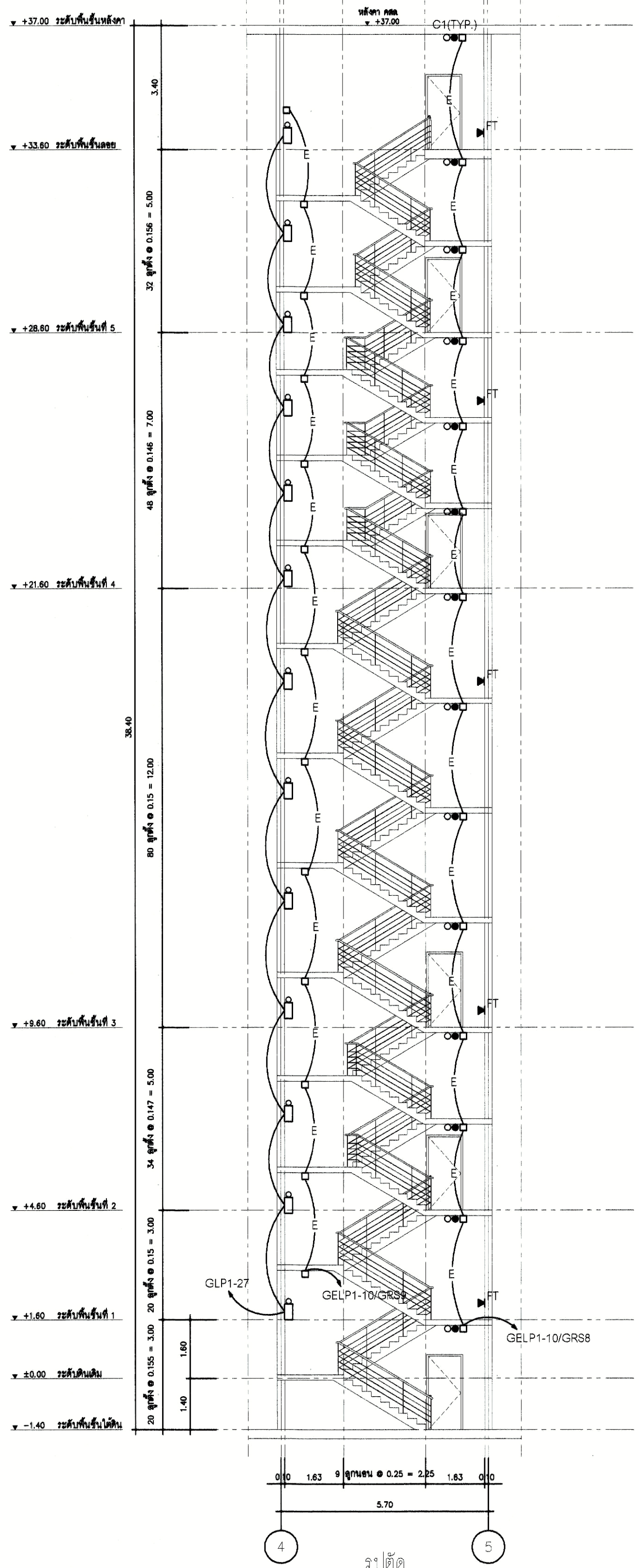
01 แบบขยายบันได ST-04
