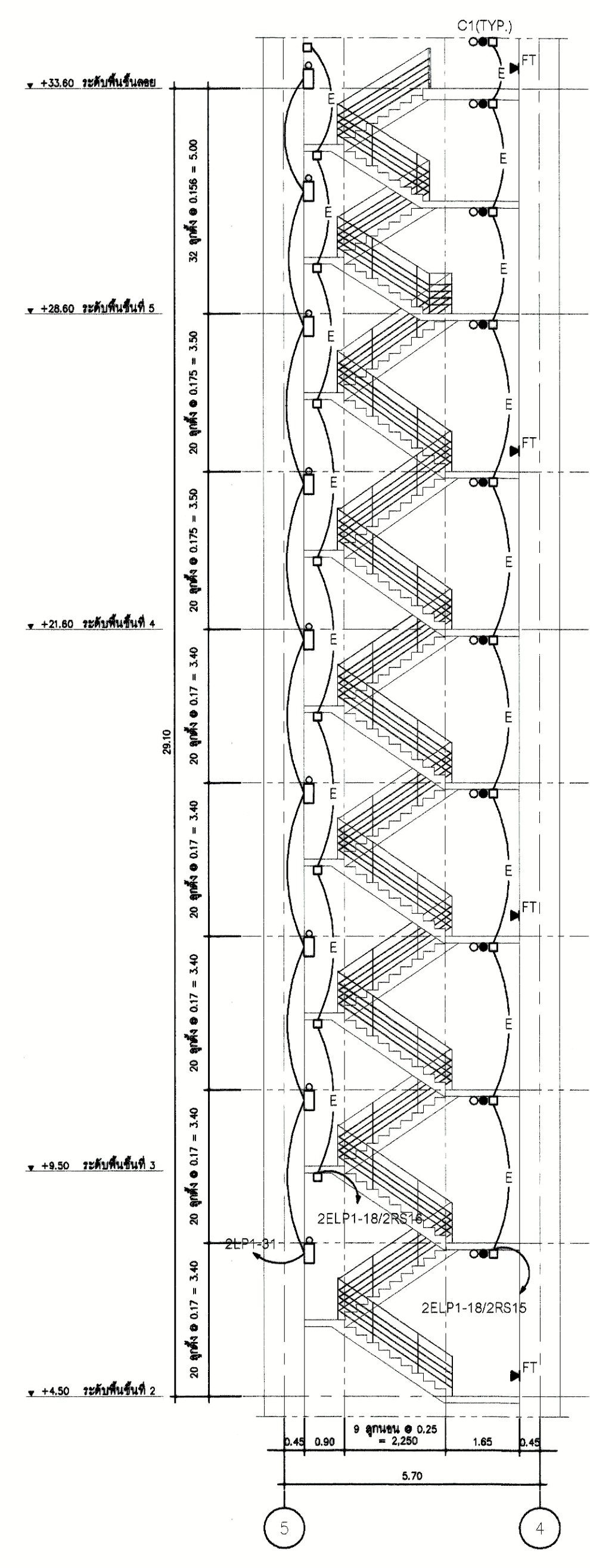
03 แบบขยายบันได ST-06
