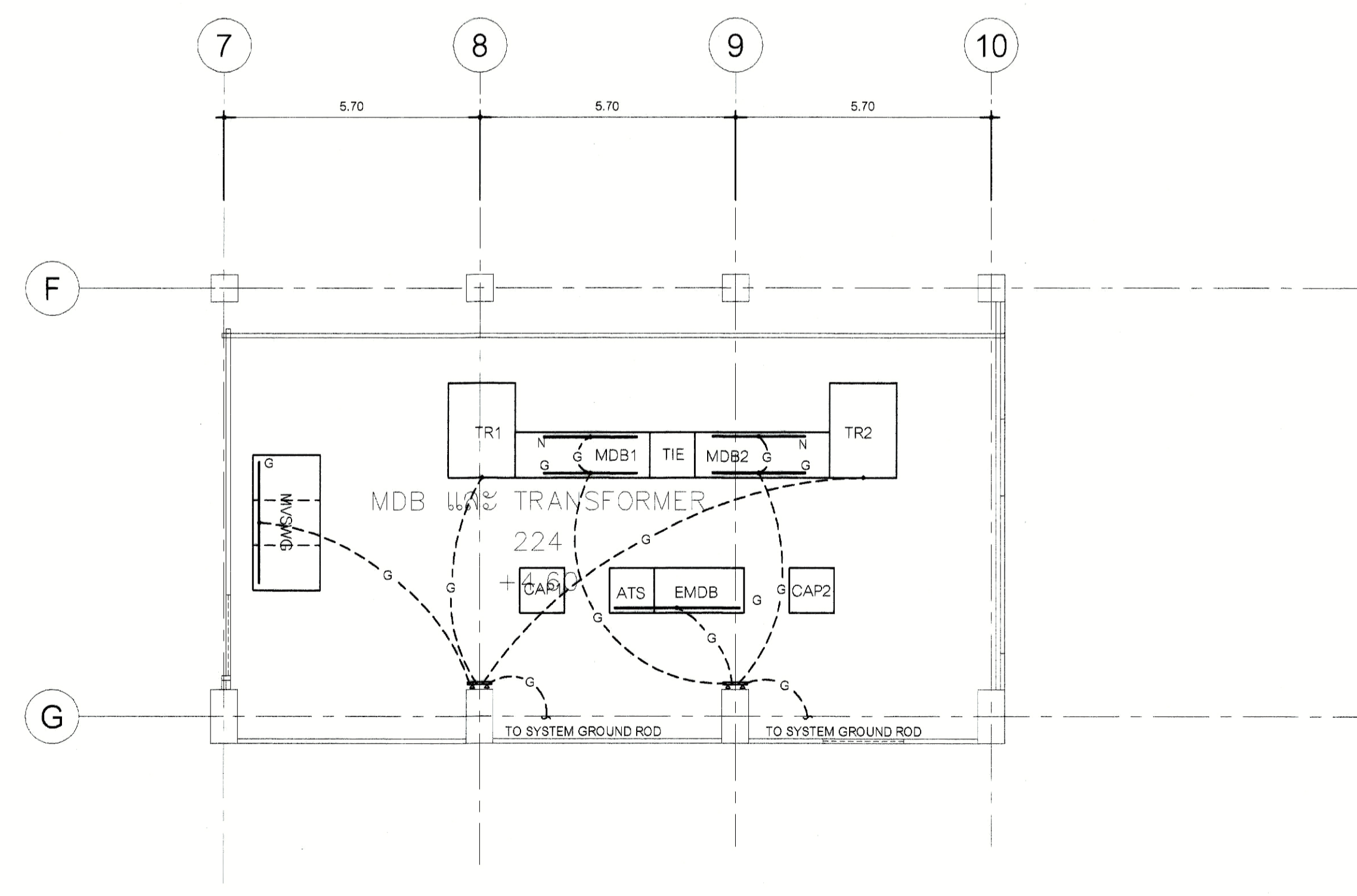
01 แบบระบบการต่อลงดินห้อง MDB
