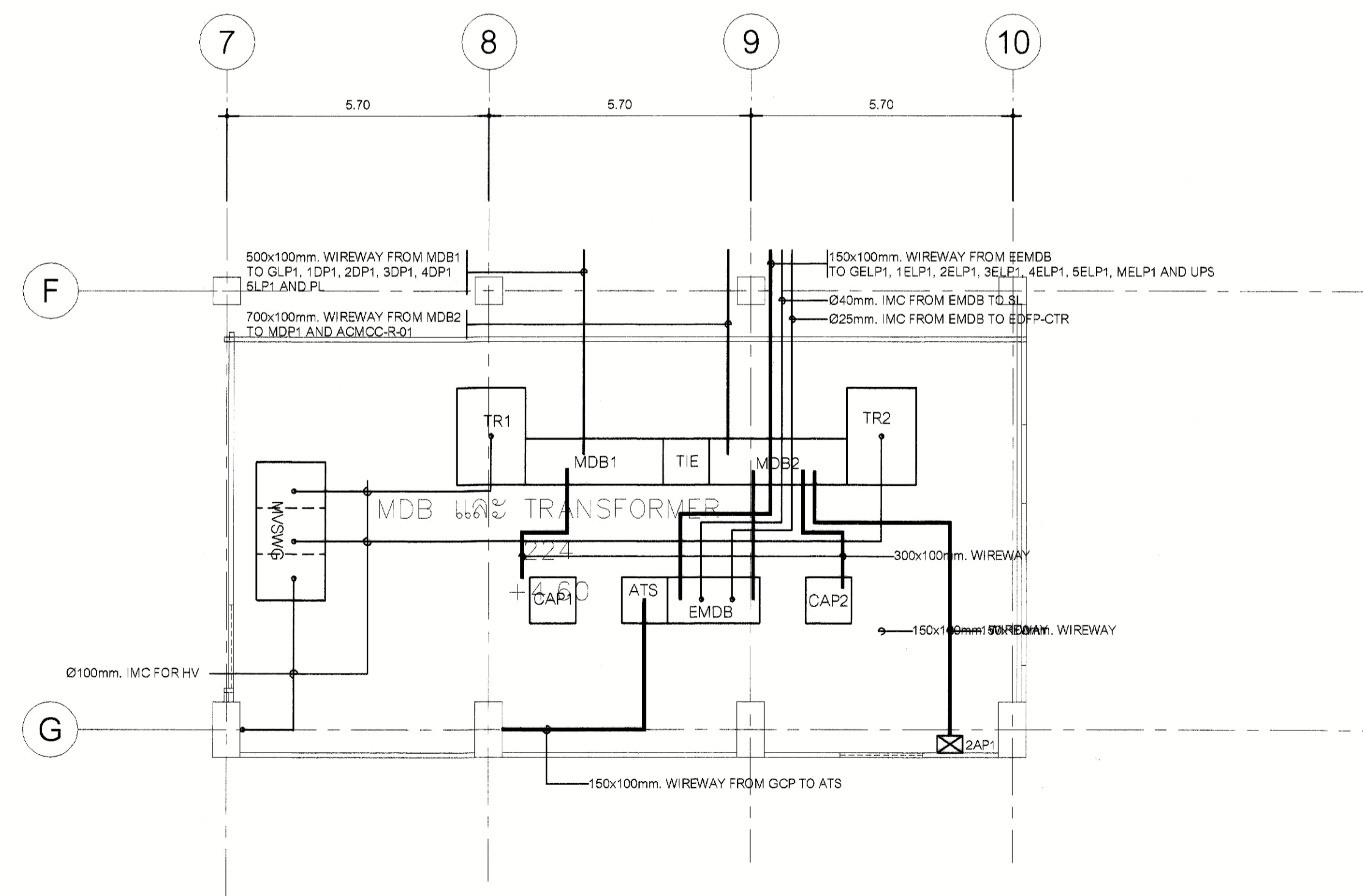
01 แบบขยายห้อง MDB
